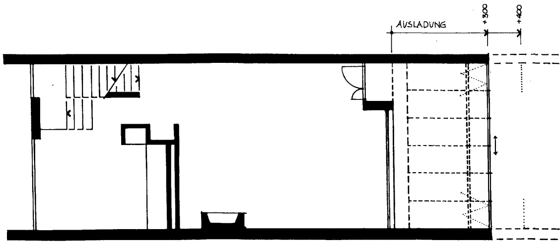
GRUNDRISS
